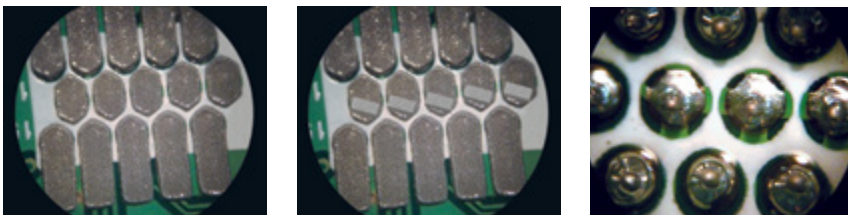
印刷后的锡膏
